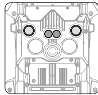
하면도
